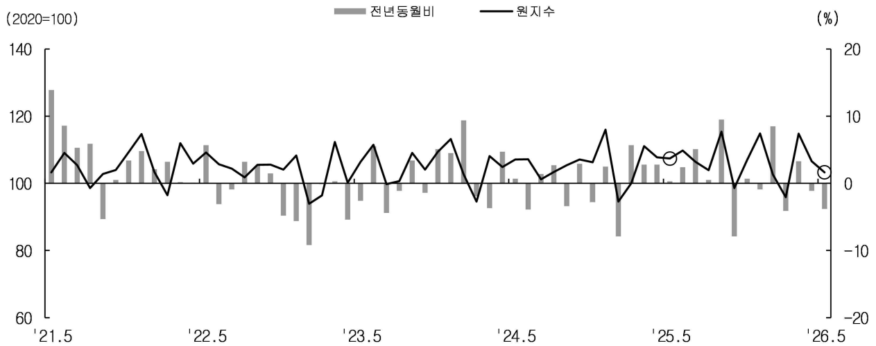
< 제조업 출하지수 전년동월비 추이 >
