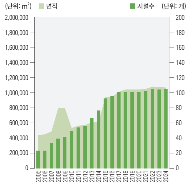
배수시설, 2005-2024
